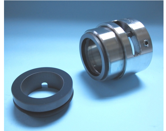
B17-R → cierre con rosca de bombeo
